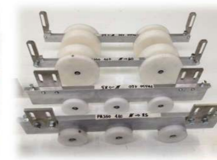
(dispositivo de cambio de paso de rodillos para gestionar diferente pasos y diferente diámetro rodillos)
